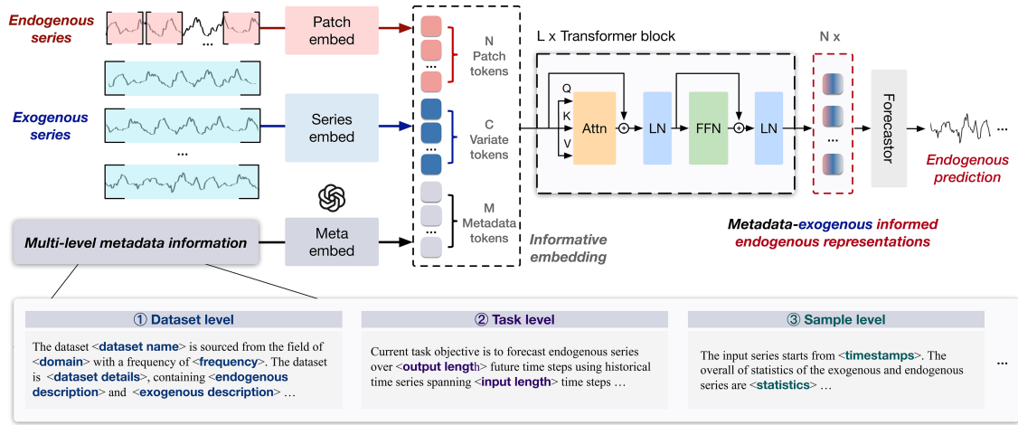
图 2 (网络版彩图) MetaTST 的整体设计. 该模型整合了内生序列、外生序列以及上下文特定的文本形式元数据, 旨在基于 Transformer 实现元数据引导的富信息时间序列预测.
