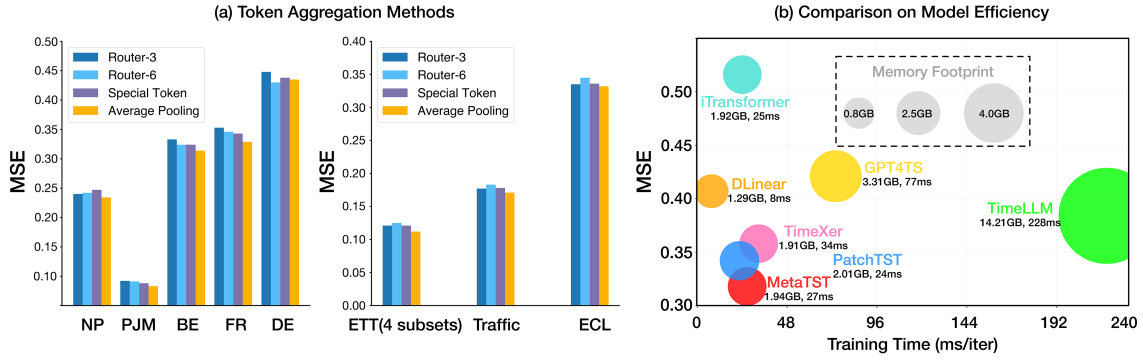
图 6 (网络版彩图) (a) 元数据词级令牌序列聚合方法有效性对比; (b) 不同模型效率比较。
