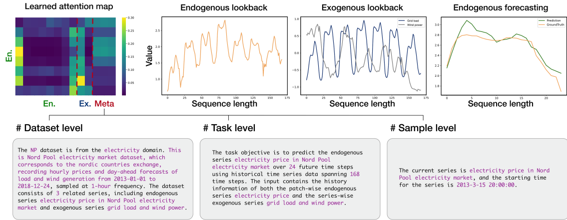
图 8 (网络版彩图) 对 NP 数据集中内生序列 (En.)、外生序列 (Ex.)、元数据 (Meta) 以及 MetaTST 中学习到的注意力分布图进行可视化。注意力分布图通过对所有注意力头的注意力矩阵进行平均计算得出。
