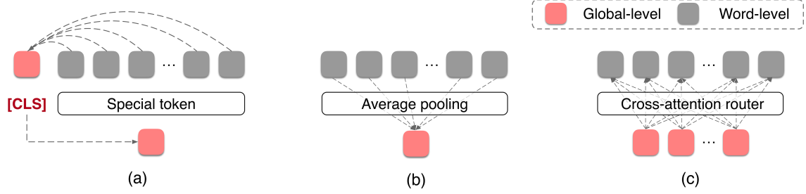
图 3 (网络版彩图) 不同的词级令牌序列到全局令牌的信息聚合方法对比, 包括 (a) 全局令牌, (b) 平均池化和 (c) 交叉注意力 3 种实现方法。
