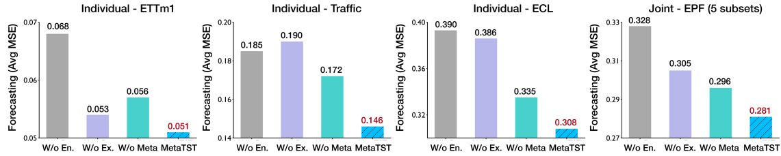
图4 (网络版彩图) MetaTST 的消融研究, 涉及富信息嵌入的不同输入信息类型, 涵盖了长、短期预测任务中的单数据集独立训练 (individual-) 和多数据集联合训练 (joint-) 策略。
