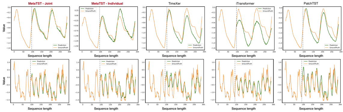
图 7 (网络版彩图) 时间序列预测案例对比, 上半部分来自于 ETTm2 数据集, 下半部分来自于 ECL 数据集。
