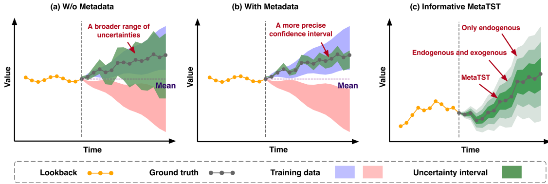
图 1 (网络版彩图) 不同时间序列预测范式的概念性对比. (a) 无元数据的经典时间序列预测范式; (b) 元数据引导的时间序列预测范式; (c) MetaTST 利用上下文特定的元数据以及协变量, 实现高确定性的富信息时间序列预测.
