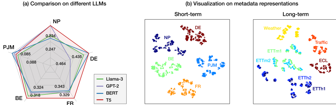
图 5 (网络版彩图) (a) 不同大语言模型作为元数据编码器的性能比较; (b) 联合训练设置下, MetaTST 在短期 (左) 和长期 (右) 预测任务下学习到的元数据表征可视化.
