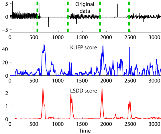
(b) HASC dataset
