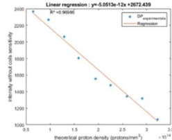
Figure 1 : Régression linéaire pour l'algorithme ESPIRiT
