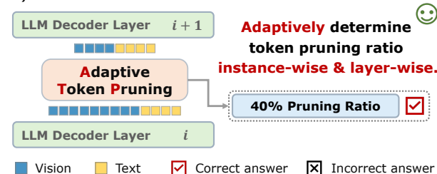
b) ATP-LLaVA.
