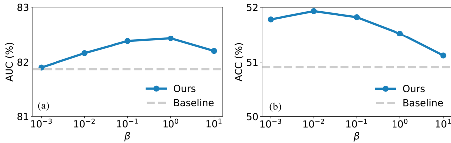
图 4 (网络版彩图) 超参数 \beta 的敏感性分析. (a) COLLAB 的结果; (b) ArXiv 的结果.
