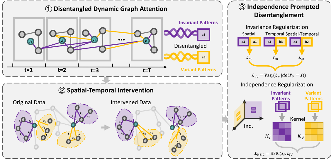
图 1 (网络版彩图) 模型框架. 所提模型主要包含 3 个模块: 解耦动态图注意力网络模块、时空干预模块和独立性促进解耦模块.
