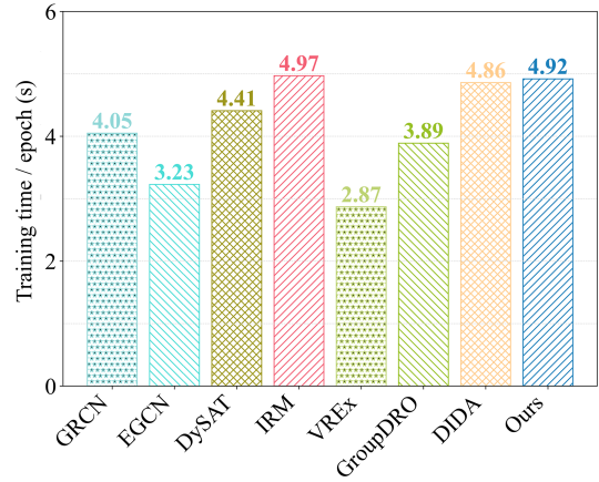
图 3 (网络版彩图) 实际时间开销比较.
