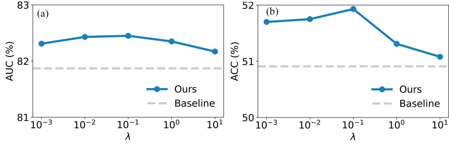
图 5 (网络版彩图) 超参数 \lambda 的敏感性分析. (a) COLLAB 的结果; (b) ArXiv 的结果.
