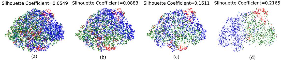
图 6 (网络版彩图) 所提方法和基线方法节点表征在 ArXiv 数据集上的可视化分析. (a) VREx 的结果; (b) GroupDRO 的结果; (c) EGCN 的结果; (d) ID-DyGAT 的结果.
