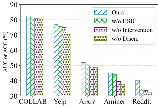
图 2 (网络版彩图) 消融实验分析.
